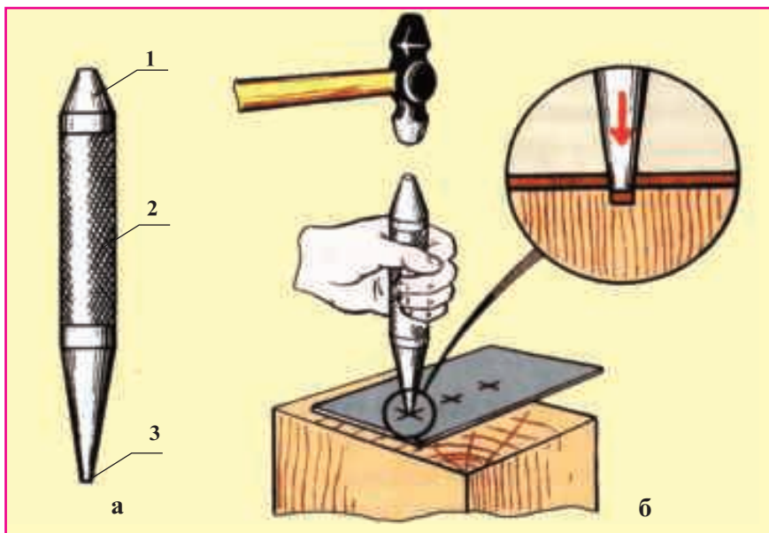
Расми 75. Сӯрох кардани металл ба воситаи сунба: а - сунба; б - раван-ди сӯрохкунӣ; 1 - ҷойи болгазанӣ; 2 - бадана; 3 - нӯғ.
