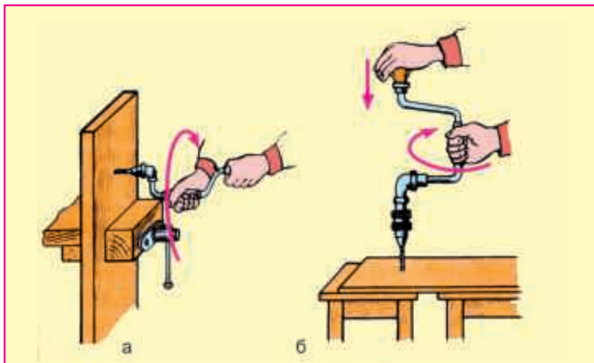
Расми 35. Тарзҳои пармакунӣ: а - дар гирои мизи дуредгарӣ; б - дар рӯйи сатҳ.
