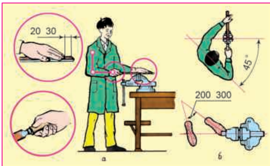
Расми 50. Ташкили кор дар мизи челонгарӣ: а - интиҳоби баландии миз; б - ҳолати дастҳо ва пойҳо ҳангоми кор.
