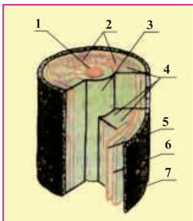
Расми 7. Буриши кундаланги танаи дарахт ва таркиби чӯб: 1 - мағз; 2 -рахҳои мағз; 3 - дила; 4 - солҳалқаҳо; 5 - камбий (парда); 6-қабати дарунии пӯст; 7 - пӯстлох.
