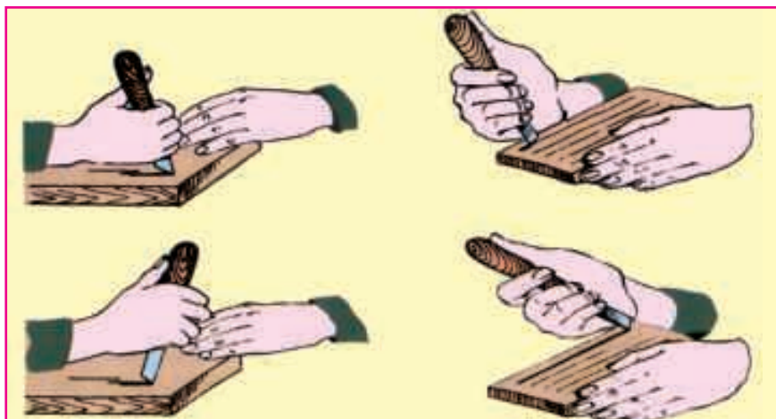
Расми 110. Тирзи дар даст нигоҳ доштани асбоби буриш ҳангоми гузоштани нақшу хатҳои ибтидоӣ.
