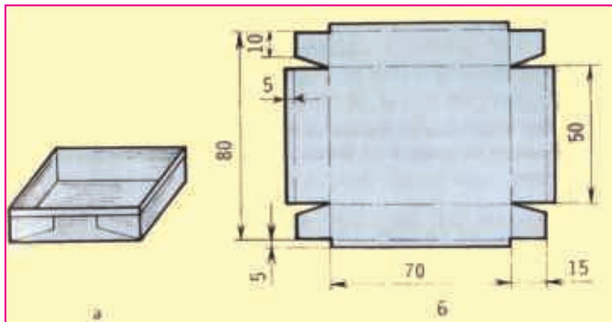
Расми 56. Маҳсулоти ҳаҷмдор аз тунука: а - расм; б - нақшаи густара.
