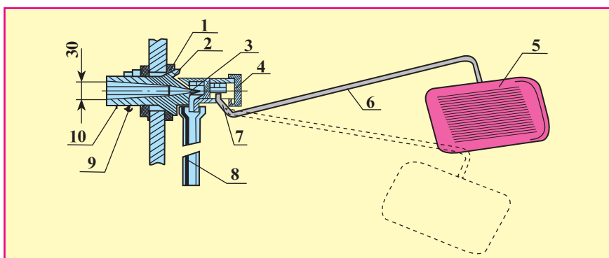
Расми 92. Қрани ғаммазакдор: 1 - прокладка; 2 - тана; 3 - пўки маҳкамкунандаи резинӣ; 4 - сарпўшак (заглушка); 5 - ғаммазак; 6 - фишанги латунӣ; 7 - тир; 8 - новачаи резинӣ; 9 - шайба; 10 - гайка.
