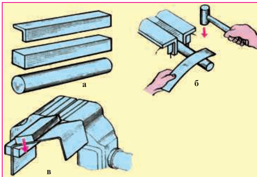
Расми 69. Қатқунии тунука ба воситаи қолабҳои металлӣ: а - қолабҳои металлӣ; б, в - тарзҳои қатқунӣ.
