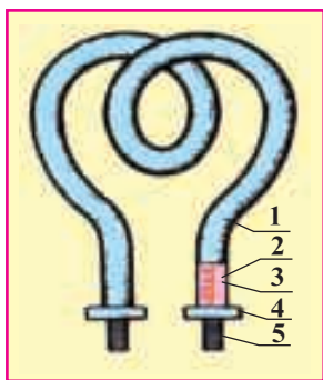
Расми 103. Ҷузви гармкунанда: 1 - қубури металлӣ; 2 - спирали гармкунанда; 3 - реҷи кварсӣ; 4 - эмали махсус; 5 - шилкаи пайвандӣ.
