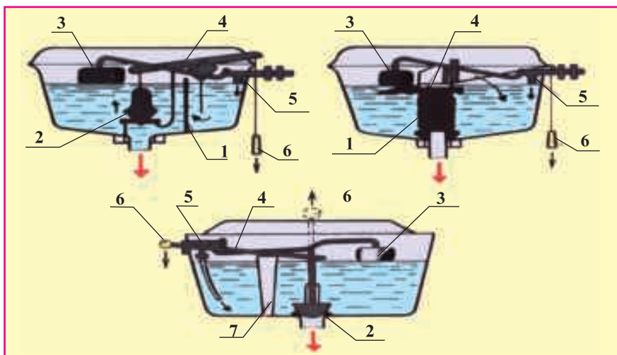
Расми 91. Сохти бакчаҳои ташиноб: а - калонҳаҷми сифонаш металлӣ; б - калонҳаҷми сифонаш резинӣ; в - хурдҳаҷм; 1 - сифон; 2 - клапани баромад; 3 - ғаммазак; 4 - фишанг; 5 - қрани ғаммазак; 6 - дастак; 7 - найчаи ҷоришавии об.
