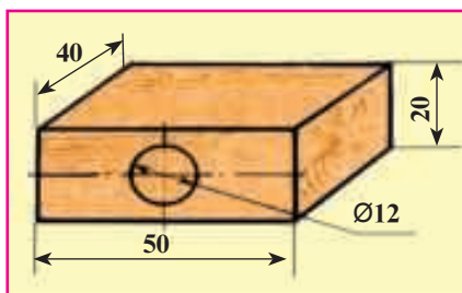
Расми 13. Расми техникӣ ҷузв (детал)
