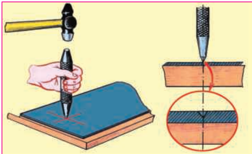
Расми 77. Нуқтагузори (аломатгузори) ҷойи сӯрохкунӣ.
