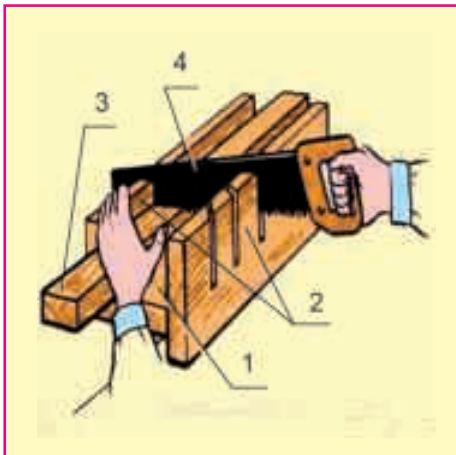
Расми 27. Арракунии бо ёрии стусло: 1- асос; 2 - девораҳо; 3 - тахтама- солех, 4 - арра.
