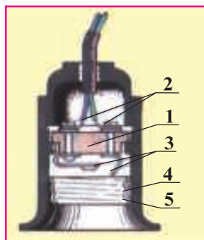
Расми 102. Патрони овезаи лампа: 1 - дила; 2 - ғироҳои винтӣ; 3 - ит- тисолҳои пружинӣ; 4 - рахпеч; 5 - бадана.
