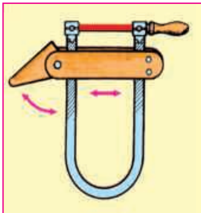
Расми 45. Вазит барои фишурдани чавкоти симарра.
