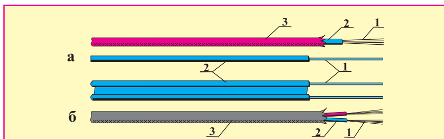
Расми 94. Симхо (ноқилҳо) (а) ва ин (б): 1 - ноқили барқгузарон; 2 — изолятсия; 3 - парда.
