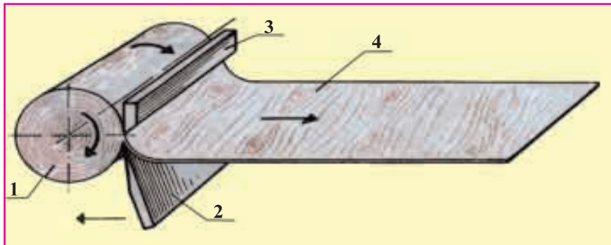
Расми 11. Схеми буридани тахтаварақ барои фанера: 1 - гӯлачӯб; 2 - теғ; 3 - ҷафсак; 4 - варақи фанера.
