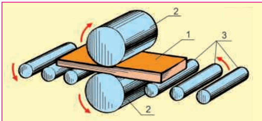
Расми 52. Схекаи ҳосил кардани тунука: 1 - моли хом ё худ масолеҳ; 2 - навардҳо; 3 - гилдиракҳо.
