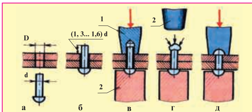
Расми 84. Марҳалаҳои пайвасткунии ба воситаи парчин: а — сӯрохкунӣ; б - ҷойгир кардани парчин; в - ҷойгир кардани маҳсулоти парчиншаванда; г - парчин кардани сарак; д - шаклдиҳии парчини сарак (1 - кашии додан; 2 - дошта истодан; 3 - болға; 4 - фишурдан).
