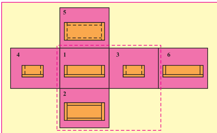
Расми 18. Шаш намуди маҳсулот. 1 - асосӣ (аз пеш); 2 - аз боло; 3 - аз чап; 4 - аз рост; 5 - аз поён; 6 - аз қафо.
