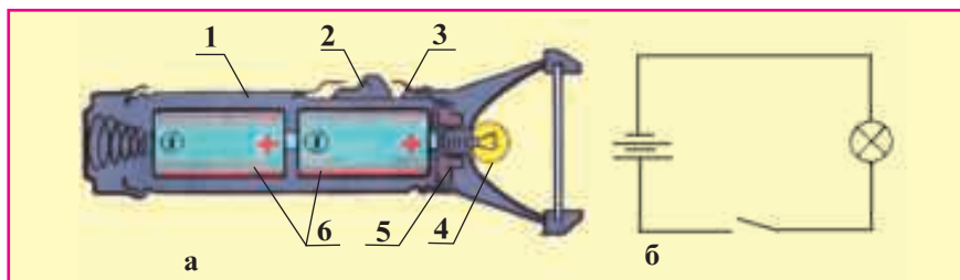
Расми 96. Сохти ҷароғи дастӣ (а) ва схемаи барқии он (б): 1 - бадана; 2 - даргиронанда ва ҳомӯшкунанда; 3 - иттисоли даргиронанда ва ҳомӯшкунанда; 4 - лампочка; 5 - изолятор; 6 - батареяҳо.
