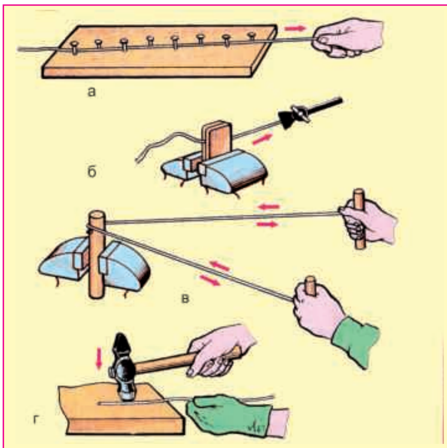
Расми 59. Рост кардани симҳо.
