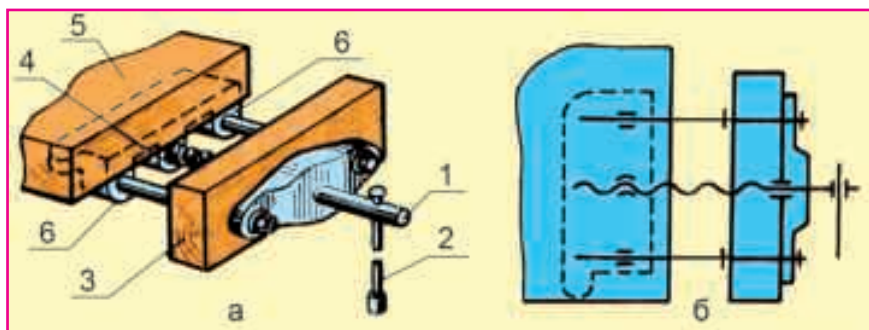
Расми 48. Ғирои винтии мизии дуредгарӣ (а) ва нақшаи кинематикии он (б): 1 - винти ҳаракатнок; 2 - даста; 3 - тахтачаи ғиро; 4 - ғайка; 5 - сарпӯши миз; 6 - тақягоҳ.
