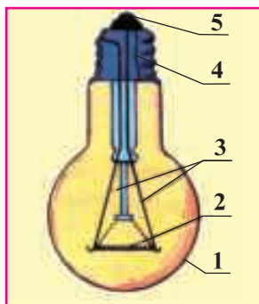
Расми 101. Соҳти лампочкаи рӯзгор: 1 - иттиҳа; 2 - муякаи тафсанда; 3 - электродҳо; 4 - печтоб; 5 - иттиҳоли марказӣ.
