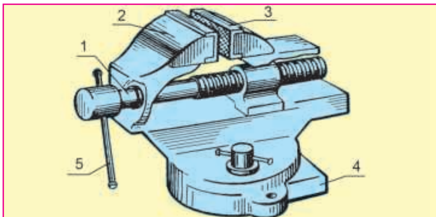
Расми 51. Шиканҷаи челонгарӣ: 1 - винти ҳаракатнок; 2 - лаби ҳаракатнок; 3 - лаби беҳаракат; 4 - лавҳачаи тақягоҳӣ; 5 - даста.
