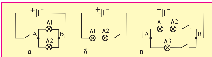
Расми 97. Тарзҳои гуногуни пайвастунии лампочкаи барқӣ ба манбаи барқ; а - мувозӣ; б - пайиҳам; в - омехта.
