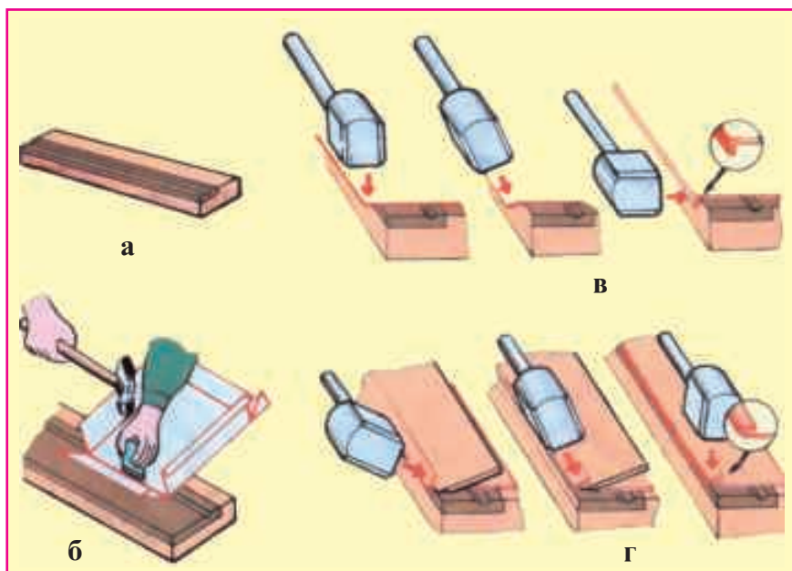
Расми 71. Қатқунии тунуқаҳои дароз: а - асбоби қатқунӣ, б, в, г - тарзҳои қатқунӣ.
