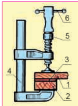
Расми 40. Шиканча: 1,2- деталҳои ширеш- шаванда; 3 - ширеш; 4 - танаи шиканча; 5 - печи шиканча; 6 - дастаи шиканча.
