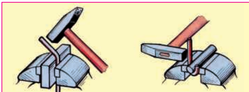
Расми 74. Қаткунии сими ғафс дар шиканча.
