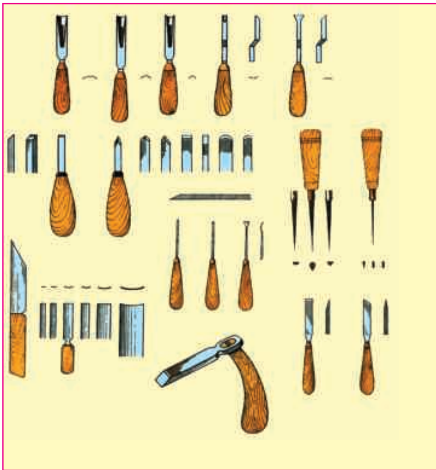
Расми 113. Исканаҳо (а) ва асбобҳо (б).
