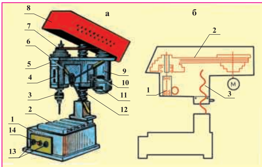
Расми 81. Дастгоҳи пармакунӣ: а - сохти умумӣ; (1 — асос; 2 - мизи корӣ; 3 - патрон; 4 - шкалаи танзими чуқурии пармакунӣ; 5 - гирои шпинделӣ; 6 - дастак; 7 - ҳаракатгузаронӣ бо тасма; 8 - рӯйкаши муҳофизатӣ; 9 - муҳаррики барқӣ; 10 - дастаи танзими гирои шпинделӣ; 11 - дастаи ба поён ҳаракатдиҳандаи гирои шпинделӣ; 12 - колонна; 13 - тугмачаҳои ба ҳаракатдарорӣ; 14 - тугмачаи “Ист”) б - схемаи кинематикӣ (1 - ҳаракатдиҳандаи рейкагӣ; 2 - ҳаракатдиҳандаи тасмагӣ; 3 - ҳаракатдиҳандаи винтӣ).
