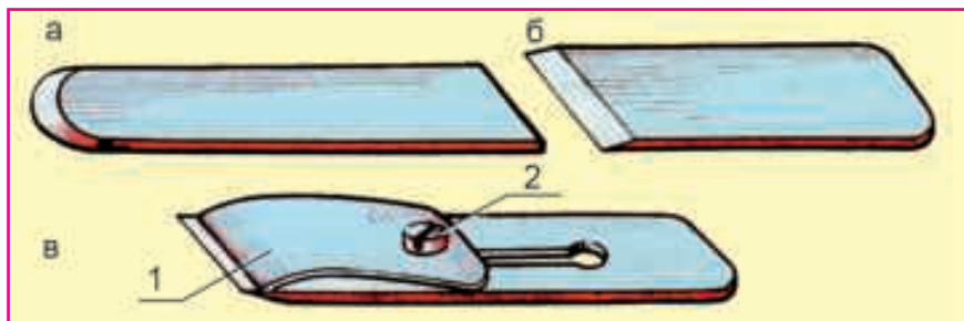
Расми 29. Тегҳо: а - теги досранда; б - рандаи одӣ; в - рандаи одӣ бо тарошашикан. 1 - тарошашикан, 2 - чархпеч.
