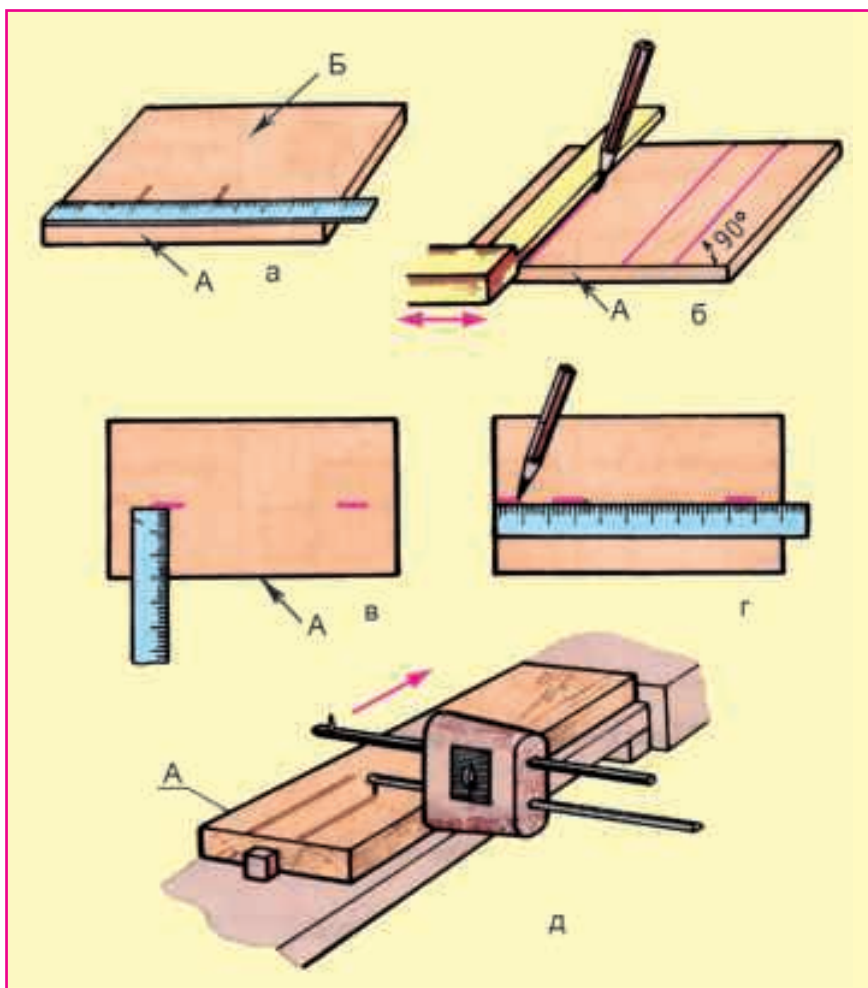
Расми 19. Аломатгузори деталҳои росткунҷашакл: а - андозагирии хатҳои мувозӣ ва амудӣ ба воситаи хаткашак; б - сабти хатҳои мувозӣ ва амудӣ ба воситаи гулӯ; в - андозагирии бари ашӯи сохтешаванда аз канораи он, яъне А; г - гузаронидани хатҳои мувозӣ ба канораҳои А; д - аломатгузорӣ бо асбоби рейсмус.
