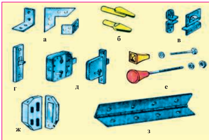
Расми 86. Фурнитураи мебел: а - кунҷакҳо; б - зермони рафҳо; в - кашакҳо; г - галақа, қулфак; д - қулфҳо; е - дастаҳо; ж - бандакҳои магнитӣ; з - ошиқ-маъшуқи роялӣ.
