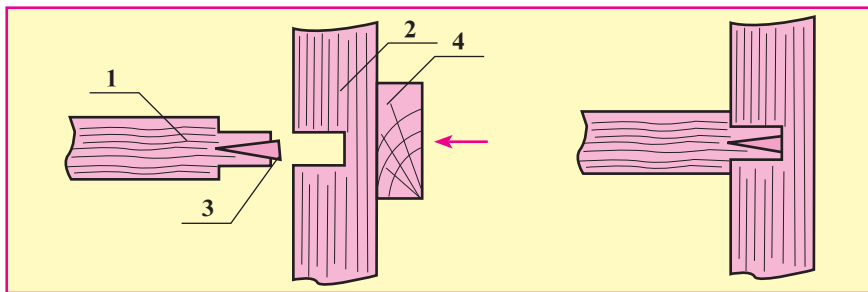
Расми 87. Схемати таъмири болочӯби ҷунбонакшудаи курсӣ: 1 - болочӯб; 2 - поя; 3 - фонача; 4 - тахтача.
