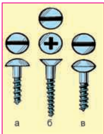
Расми 37. Рахпечҳо: а - сараки нимқуррадор; б - ниҳоншаванда; в-нимниҳоншаванда.
