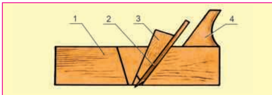
Расми 30. Сохти рандаи одӣ: 1 - асос ё худ тана; 2 - тег; 3 - фона; 4 - даста
