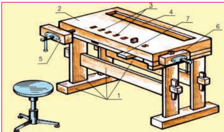
Расми 4. Мизи дуредгарӣ: 1 - асос; 2 - сарпӯш; 3 - сӯрохиҳо барои фона; 4 - нова; 5 - гирои пеш; 6 - гирои қафо; 7 - ангуштҳои ҳаракатнок.
