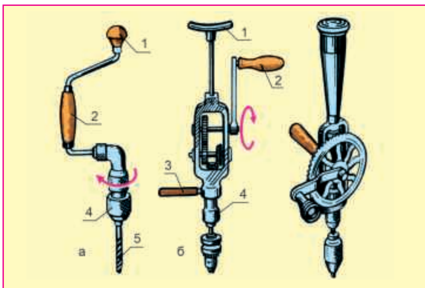
Расми 34. Асбобҳои пармакунӣ: а - шутургардан; б - парма; 1 - тақягоҳ; 2 - дастии тобдиҳӣ; 3 - дастии устуворгирӣ; 4 - патрон; 5 - парматеғ.
