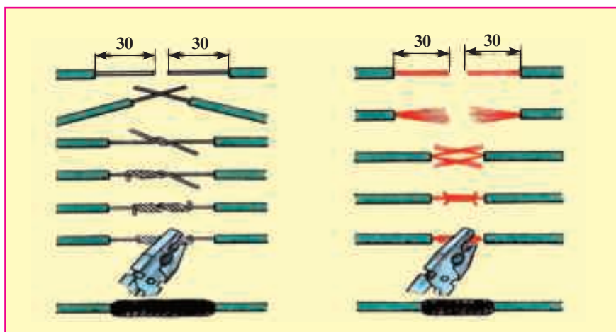
Расми 106. Тармими ноқили кандашуда.
