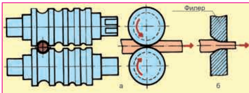
Расми 54. Схемати ҳосил кардани сим: а - ба воситаи наварди чӯякдор; б - ба воситаи филер - детали сӯрохидор.
