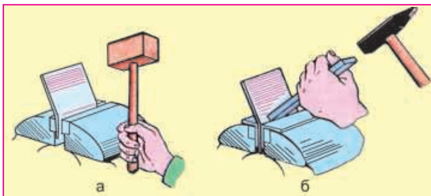
Расми 68. Қаткунии тунука дар шиканча: а - бо болғаи чӯбин; б — бо болғаи челонгарӣ ва тахтачаи чӯбин.
