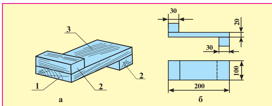
Расми 108. Сомон-олоти аррақунӣ: а - расми техникӣ (1 - асос; 2 - тақяғох; 3 - меҳи 3x4 мм) ва б - нақша.
