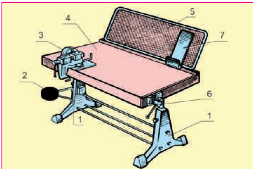
Расми 49. Мизи челонгарии универсалӣ: 1 - асос; 2 - қойи нишаст; 3 - шиканҷаи челонгарӣ; 4 - сарпӯш; 5 - симтӯри муҳофизатӣ; 6 - гирои миз; 7 - қойи гузоштани ҳуҷҷатҳои техникӣ.
