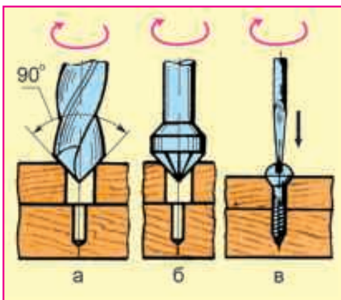
Расми 38. Тайёр кардани чойи сараки рахпеч: а - бо парма; б - бо зенковка; в - тоб додани рахпеч бо печкаш (отвёртка).
