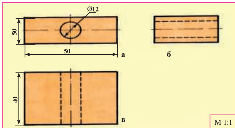
Расми 15. Нақшаи ҷузв-детал: а - намуди асосӣ; б - намуд аз паҳлу; в - намуд аз боло.
