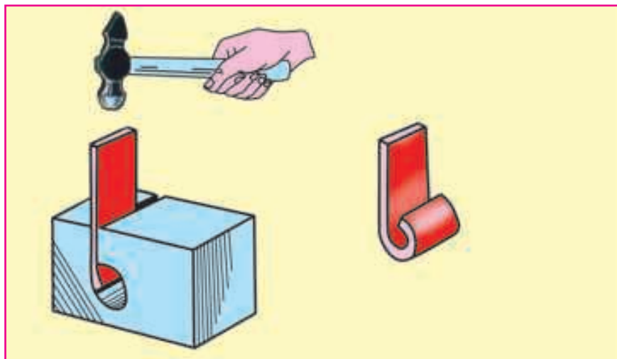
Расми 70. Асбоб барои қатқунӣ.
