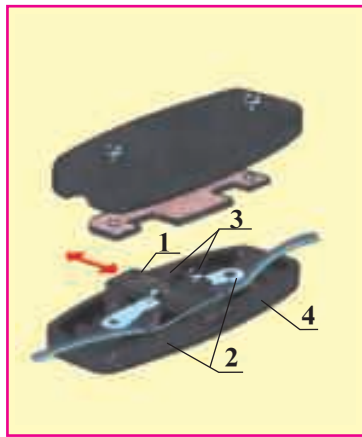
Расми 102. Сохти калиди барқӣ: 1 - иттисоли ҳаракатнок; 2 - иттисоли беҳаракат; 3 - меҳпечи фишуриш; 4 - бадана.
