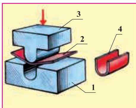
Расми 72. Қатқунӣ ба воситаи қолаб: 1 - матриса; 2 - ашғи хом; 3 - қолаб-пуансон; 4 - маҳсулоати тайёр.
