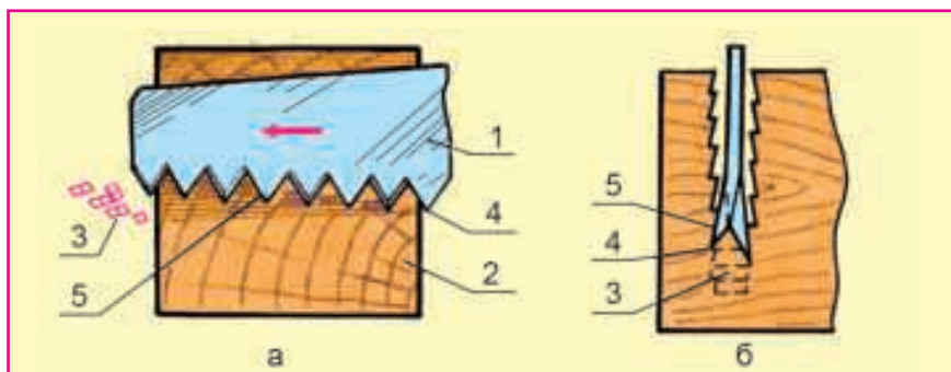
Расми 24. Буриши кундаланг: а - намуд аз паҳлуи арра; б - намуд аз буриш: 1 - арра; 2 - масолеҳ; 3 - аррамайда; 4 - нӯги дандони арра; 5 - тегаи бурандаи дандони арра
