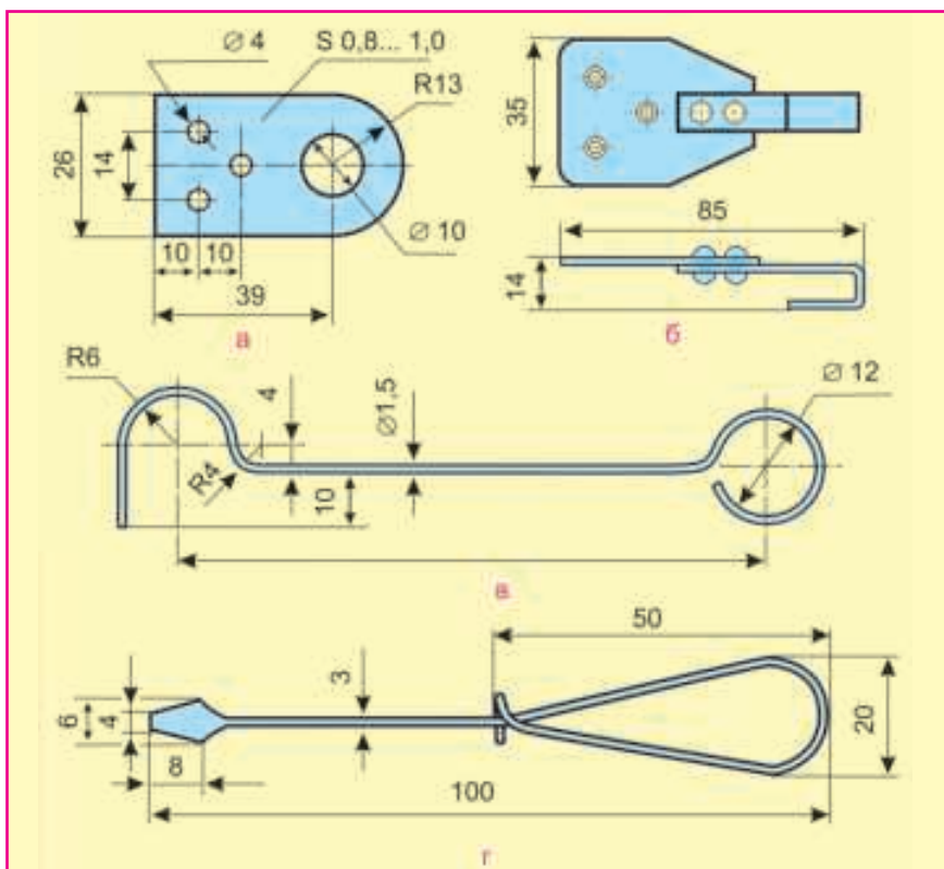
Расми 55. Нақшаи маҳсулот аз металл: а - зулфин; б - чангаки либосовезак; в - чангаки дар; г - печкаи.
