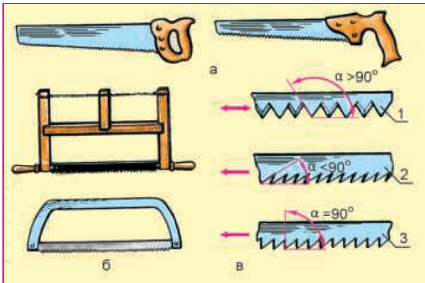
Расми 23. Намудҳои арра: а - дастарраҳо; б - камонарраҳо; в - дандонаи арраҳо. 1 - дандонаҳо барои арракунии кундаланг; 2 - дандонаҳо барои арракунии ба дарозӣ, барқад; 3 - дандонаҳо барои арракунии ҷарҳела.
