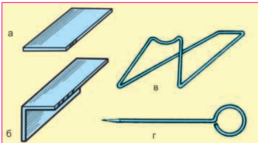
Расми 57. Маҳсулот аз тулука ва сим барои супориши 1: а - зермон-теги дастгоҳи харротӣ; б - рӯйкаши гироҳо; в - зермони кафшер, г - хаткаш.
