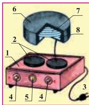
Расми 104. Плитаи барқӣ: 1 - тана; 2 - гармкунаки барқӣ; 3 - ноқили барқӣ бо вилка; 4 - калиди ивазкунии дараҷаҳои гармӣ; 5 - лампочка; 6 - асоси ҷӯяний; 7 - унсури гармкунандаи қубурӣ; 8 - қабати гарминигеҳдоранда.
