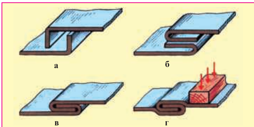
Расми 82. Пайдарпайии ҳосил кардани қатпайванд.
