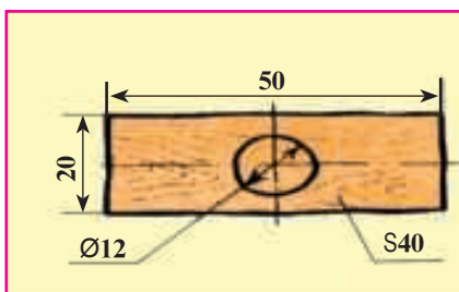
Расми 14. Ангораи ҷузв (детал).
