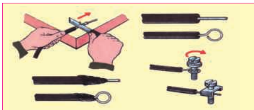
Расми 107. Пайиҳамии ҳалқакуний ва пайвасткунии симҳо
