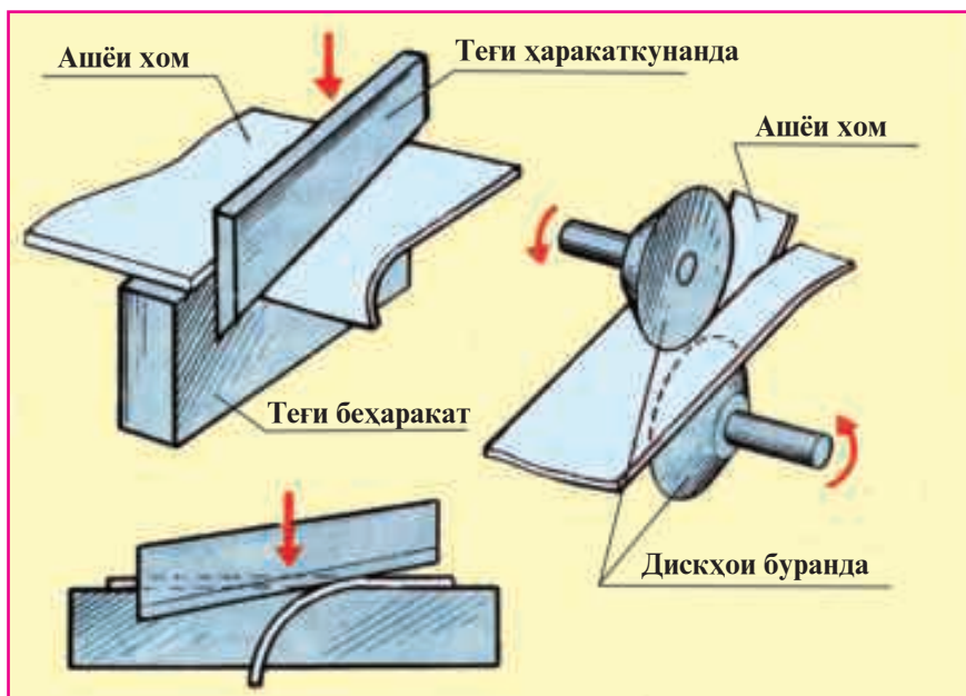
Расми 66. Буридани тунука бо қайчиҳои механикӣ: а - гилотинӣ ва б - чархӣ.
