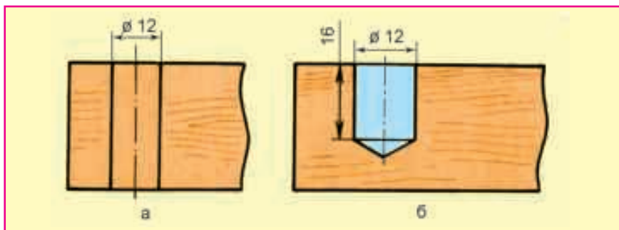
Расми 32. Сҷохиҳо: а - пурра; б - нима.
