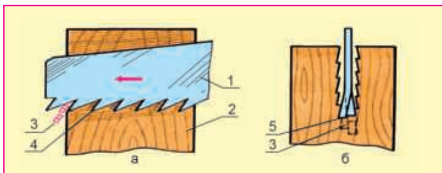
Расми 25. Буриши барқад: а - намуд аз паҳлу, б - намуди буриши арра; 1 - арра, 2 - масолеҳ, 3 - аррамайдаҳо, 4 - нӯги дандона, 5 - тегаи бурандаи дандона.
