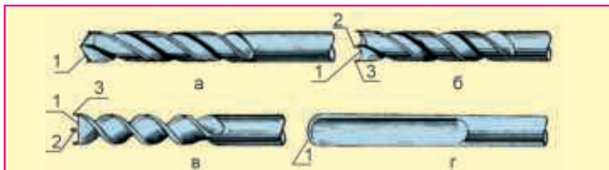
Расми 33. Парматег: а - спиралшакл; б - марказдор; в - шнекшакл, г - қошуқшакл (1 - теги пармакунӣ; 2 - марказ; 3 - зертег).
